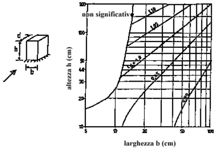
Fig C.7.10. (b) - Edifici a struttura in acciaio
