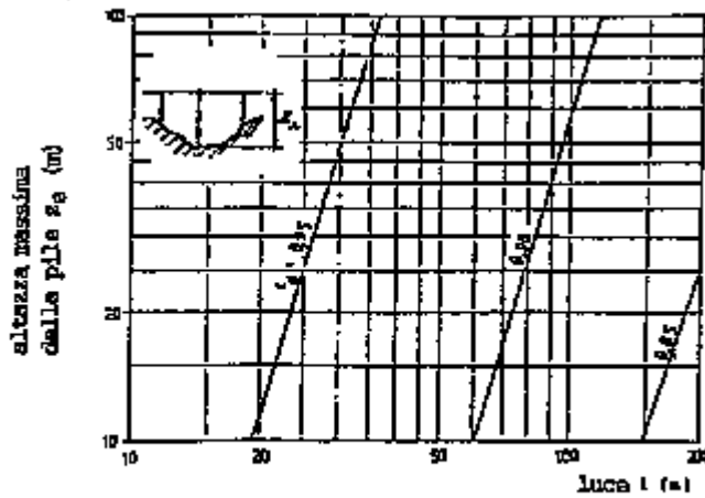
Fig C.7.12 - Ponti stradali, ferroviari e pedonaliEM>
