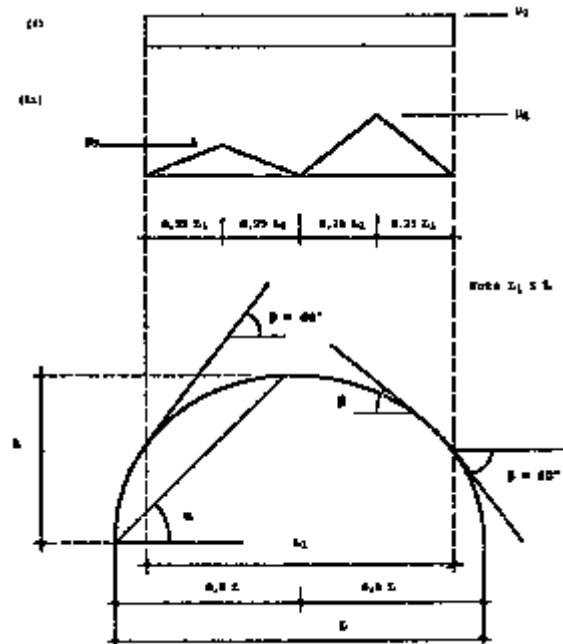
Fig C.6.6 - Coefficienti di forma per coperture cilindriche
