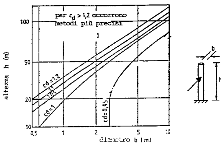
Fig C.7.11. (a) - Ciminiere in acciaio, saldate, senza rivestimento interno
