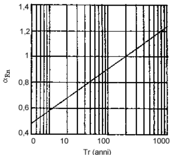
Fig C.6.11 - Valori del carico neve al suolo in funzione dell'intervento di ritorno.
