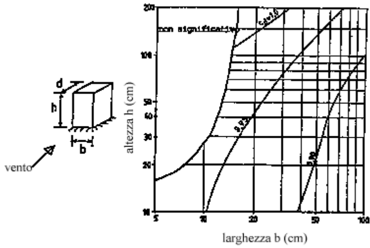
Fig C.7.10. (a) - Edifici in c.a. o in muratura
