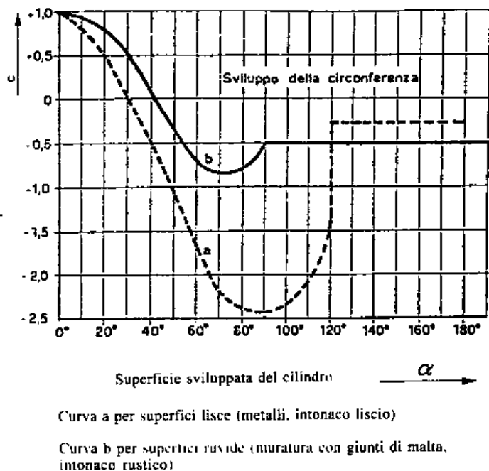
Fig C.7.9 - Coefficienti di forma c
